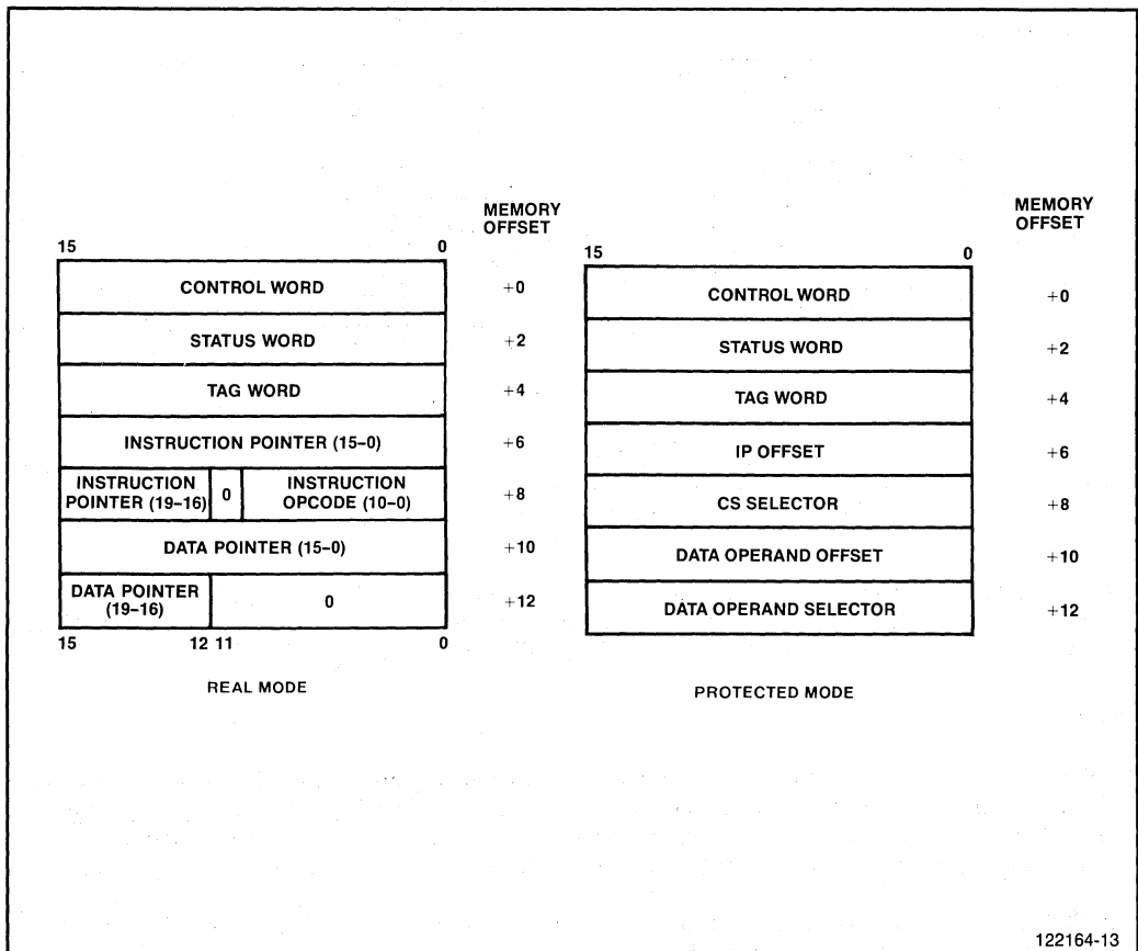
Figure 2-2. FSTENV/FLDENV Memory Layout
