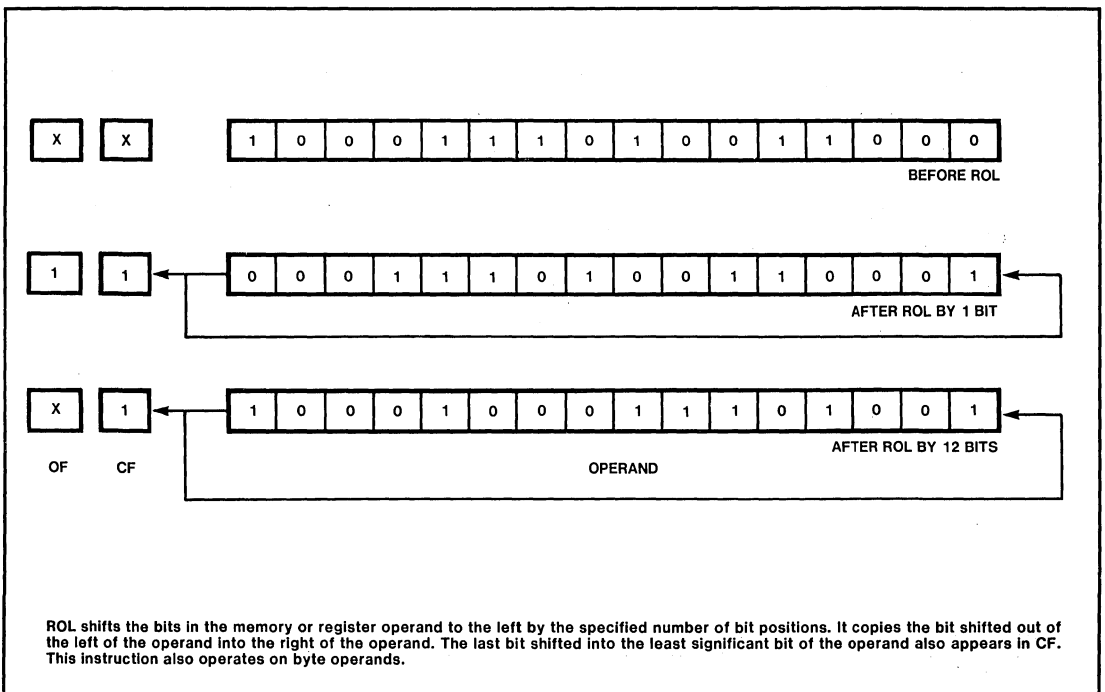
Figure 3-9. ROL
